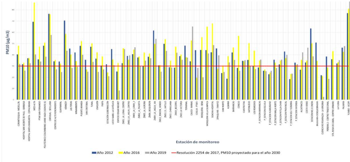
Gráfico 35. Concentración anual de material particulado (PM10, \mu\text{g}/\text{m}^3 ) por estación de monitoreo. Colombia, 2012, 2016 y 2019
